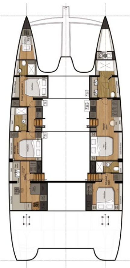
HULLS COQUES
